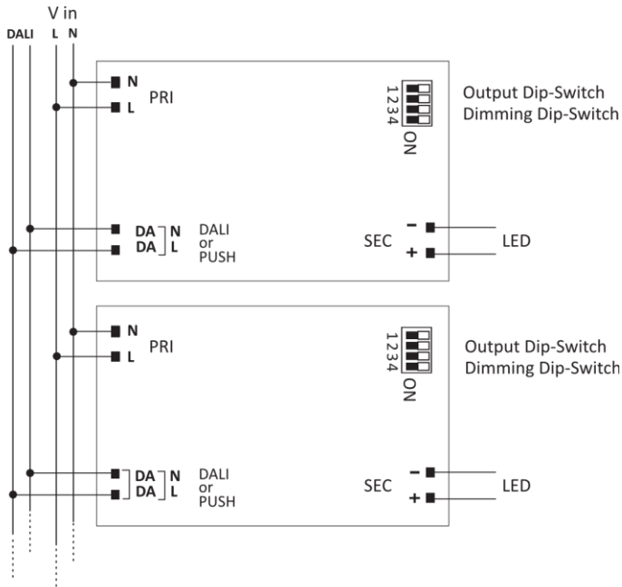
Schema di collegamento DALI, Wiring diagram DALI
